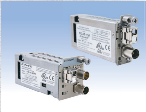
3G-SDI EO Converters
