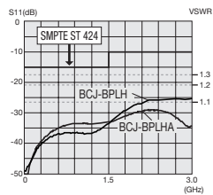
Return loss for BCJ-BPLH, BCJ-BPLHA
