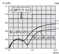
Return loss for BCJ-BPLH2P, BCJ-BPLH2PA
