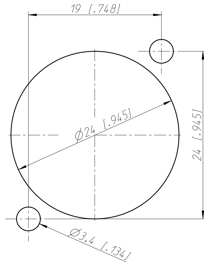
Print-Bohrplan (Bestückungsseite)
