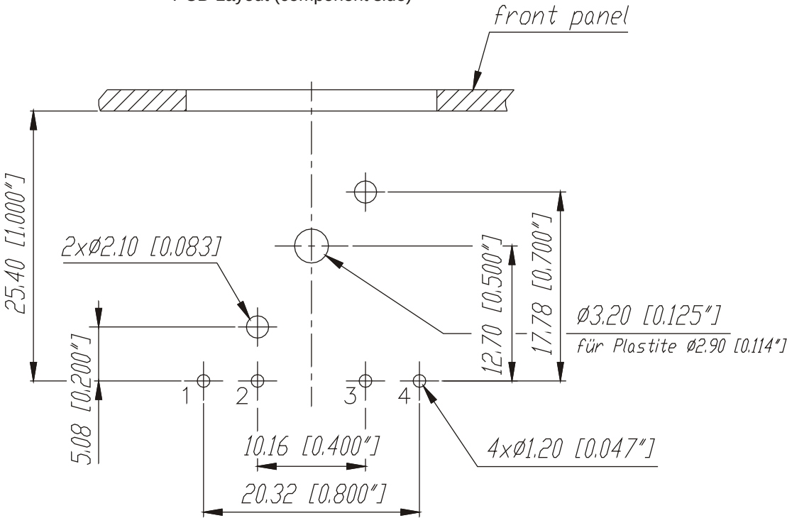
Print-Bohrplan (Bestückungsseite) PCB-Layout (component side)
