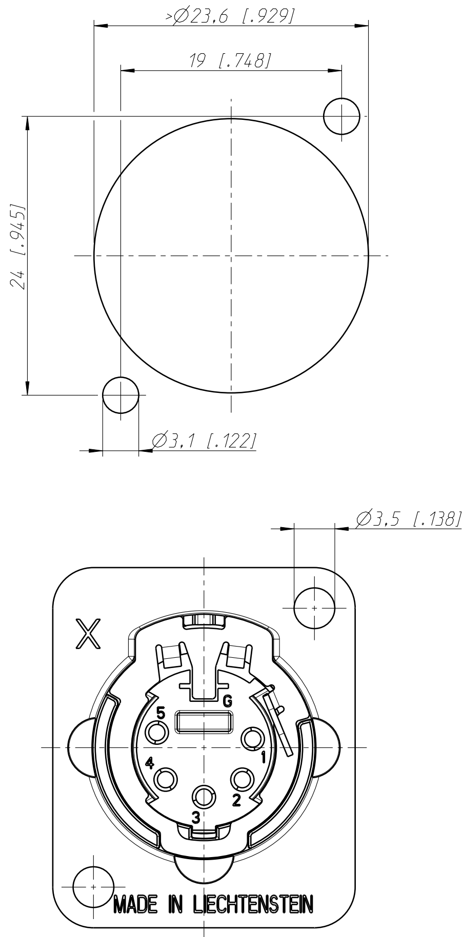
Frontplattenausschnitt (Rückseite) panel cut out (rear side)
