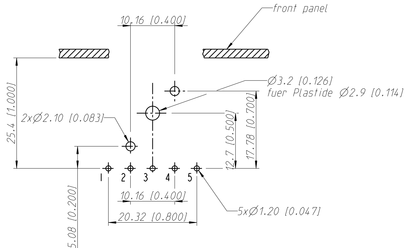
Print Bohrplan (Bestueckungsseite) PCB-Layer (component side)
