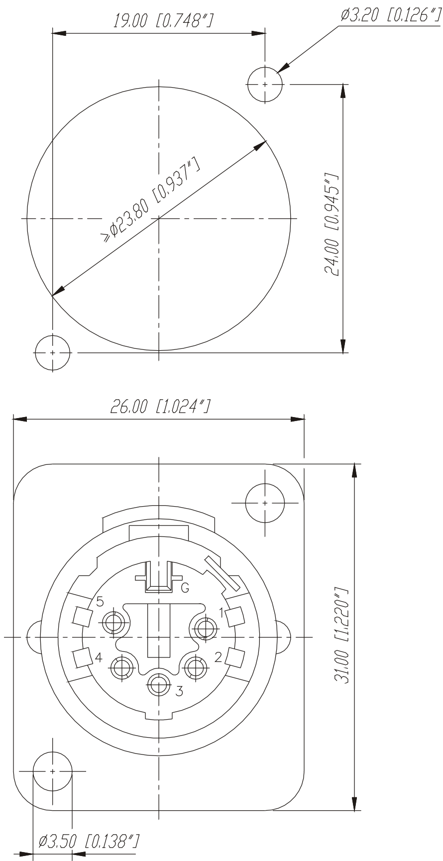
Frontplattenausschnitt (Rückseite) Panel cut out (rear side)
