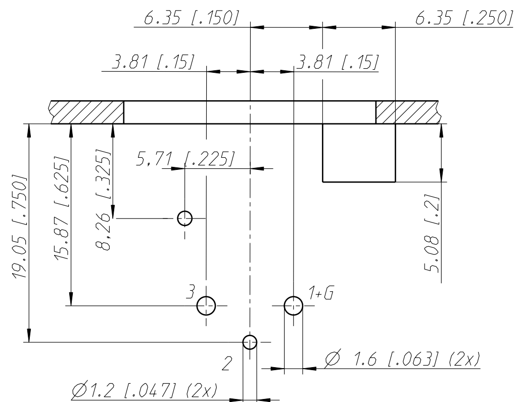
Print-Bohrplan (Bestückungsseite) PCB-Layer (component side)
