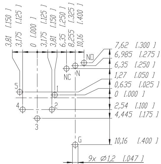
Print Bohrplan (Bestückungsseite) PCB-Layout (component side)
